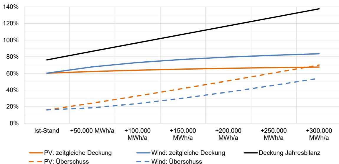
Abbildung 7.5: Deckungsanteile (jahresbilanziell und zeitgleich) sowie anteilige Stromüberschüsse im Verteilnetz des Betrachtungsraumes bei angenommenem Zubau von Strom aus PV- oder Windkraftanlagen
