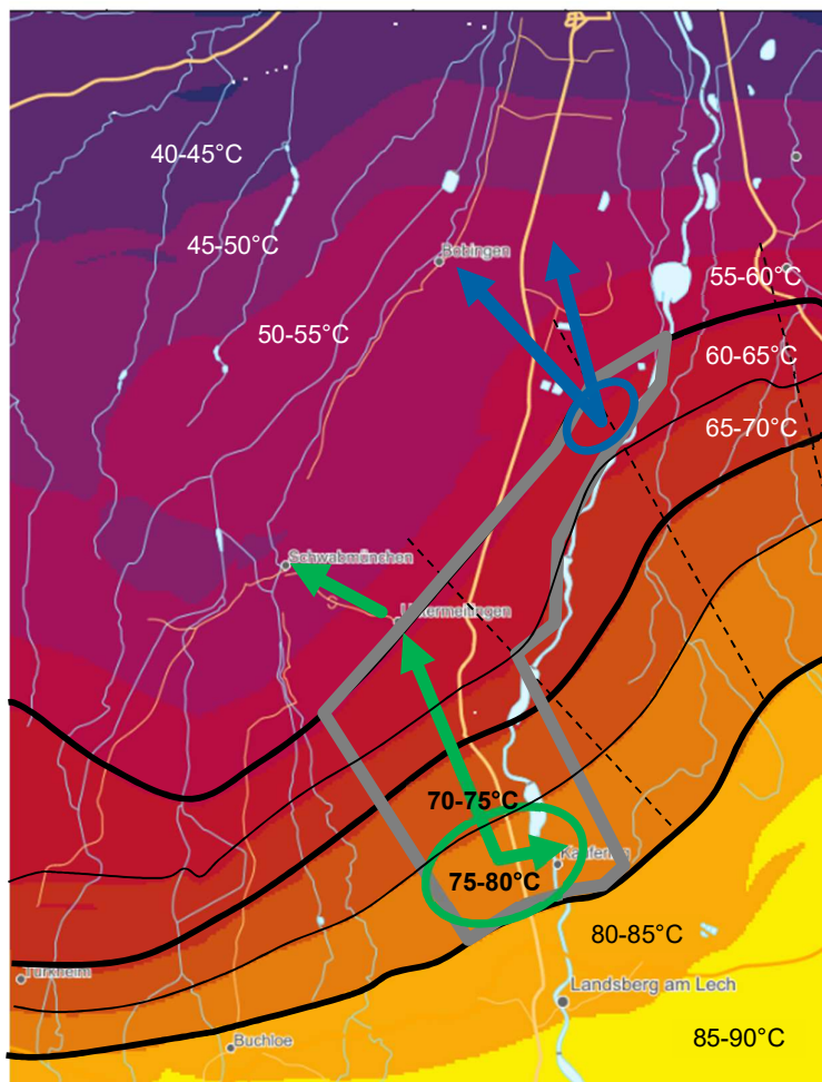
Abbildung 7.11: In Betracht gezogene Aufsuchungszonen (blaue/grüne Kreise) und mögliche Erschließungspfade (blaue/grüne Pfeile) der Geothermie. Identifikation auf Basis der Isothermen (schwarze Linien) auf Niveau des Malms im herausgearbeiteten Untersuchungsgebiet (graue Umrandung). Hintergrundkarte: Horizontalschnitt, Malm (GeotIS, 2024)
