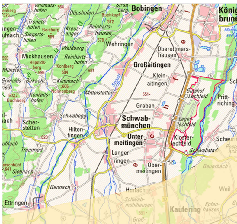
Abbildung 4.7: Eignungsgebiete für hydrothermale Wärmegewinnung (LfU, 2024 b) ■ Günstige geologische Verhältnisse für hydrothermale Wärmegewinnung ■ Weniger günstige Verhältnisse für hydrothermale Wärmegewinnung (i.d.R. zusätzlicher Wärmepumpeneinsatz erforderlich)
